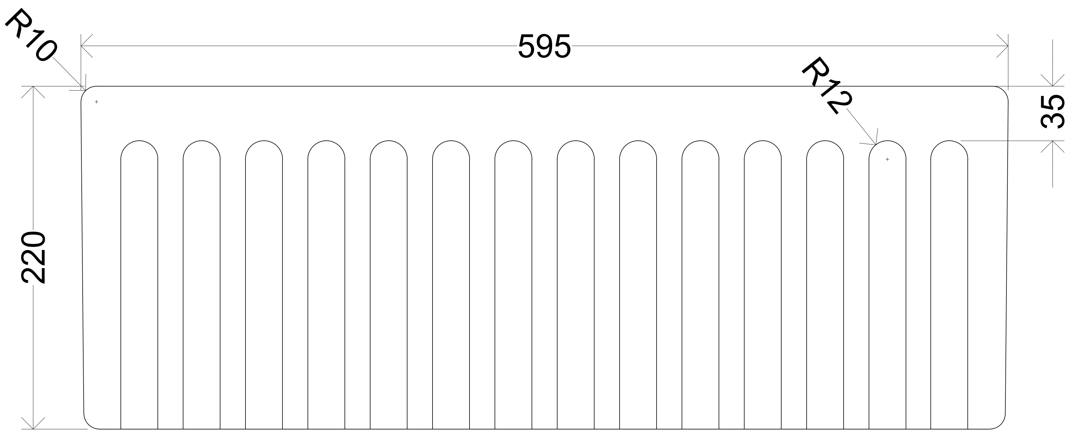
ELEVATION
